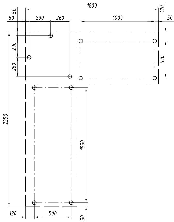
Рис.3 Точки крепления изделия к палубе
