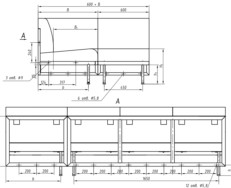
Рис. 2 локотники съемные остальное см. рис. 1
