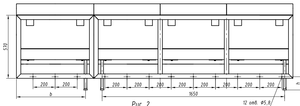
Рис. 2 локотники съемные остальное см. рис. 1
