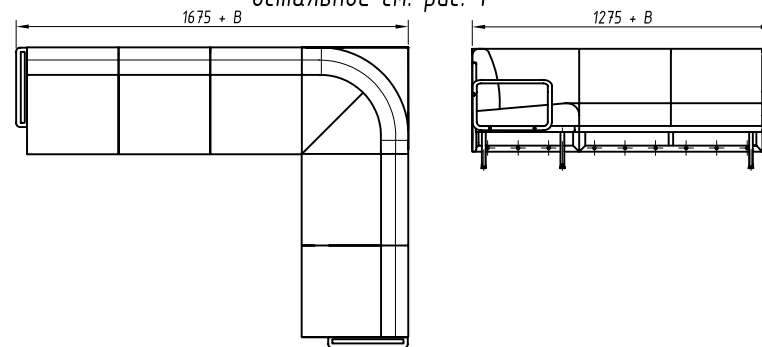
Рис. 2 локотники съемные остальное см. рис. 1
