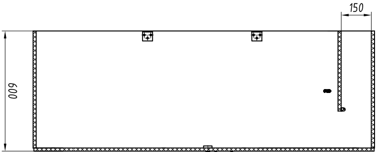
Рис. 1 А-А
