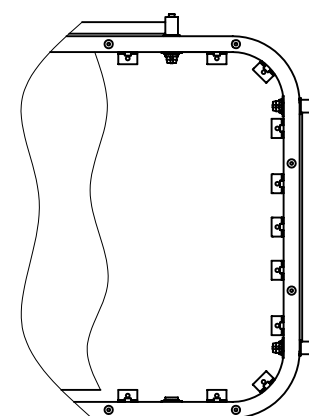
Рис.2 Рама с жестким основанием
