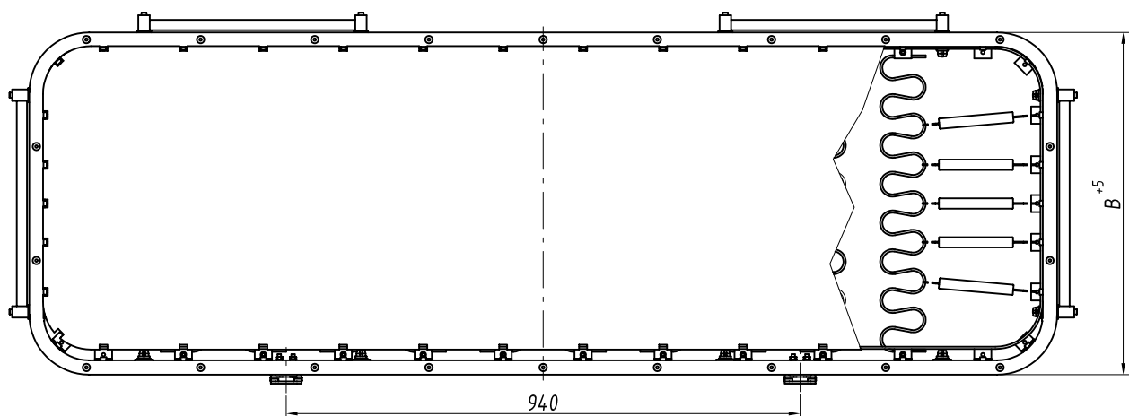
Рис.1 Рама с волнообразными пружинами
